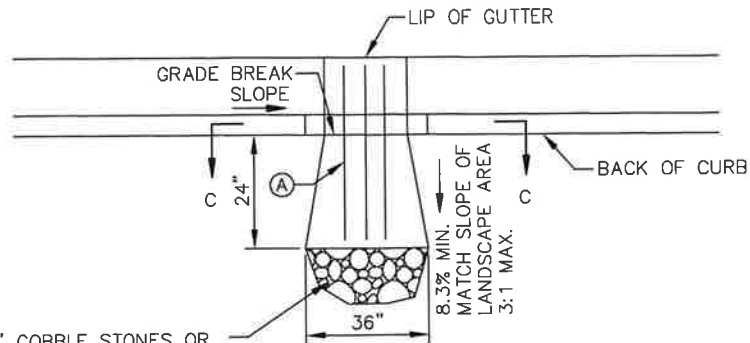
PLAN N.T.S.
